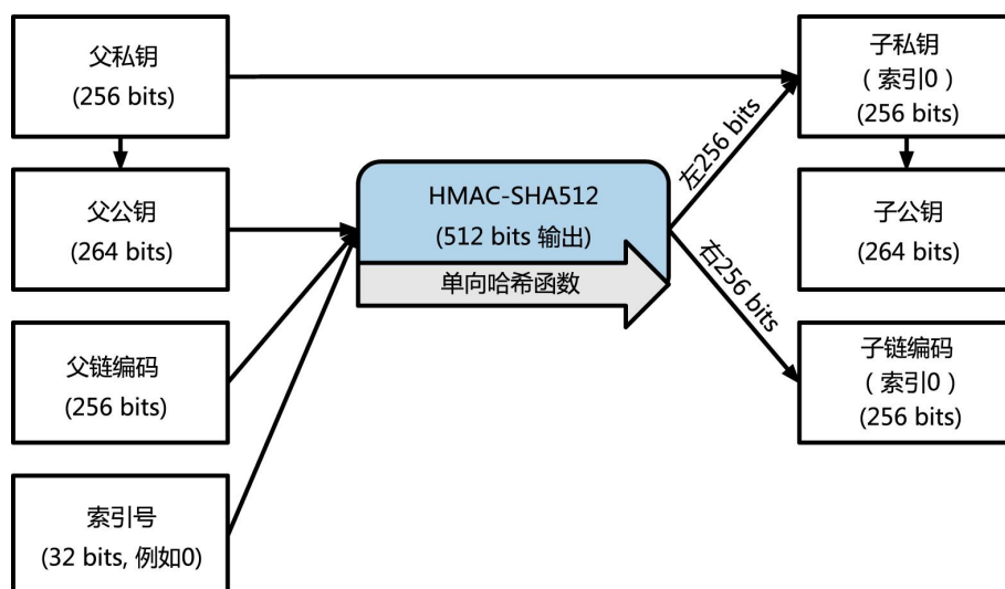
图 4-11 延长母私钥去创造子私钥
