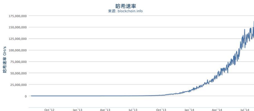
图 8-7 近两年的总算力，G 次 hash/秒
