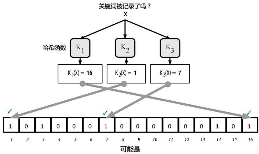
图 6-11 验证关键词 “X” 是否存在于 Bloom 过滤器中。
