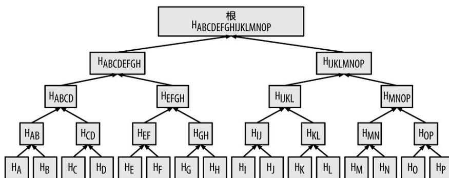
图 7-4 一颗囊括了许多数据元素的 Merkle 树
